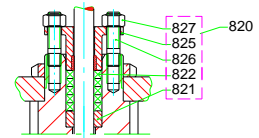
DN 80-100, PN 16-40
