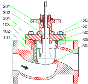
MV 5211, PV 6211 mit/ with/ avec QCS DN 80 – 100, PN 16 – 40
