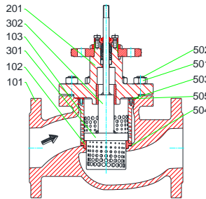
MV 5211, PV 6211 mit/ with/ avec QCS 2-stage DN 80 – 100, PN 16 – 40
