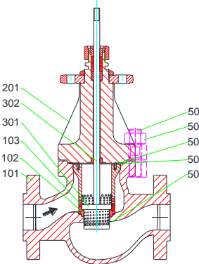
MV 5211, PV 6211 mit/ with/ avec QCS 2-stage DN 15 – 50, PN 63 – 100
