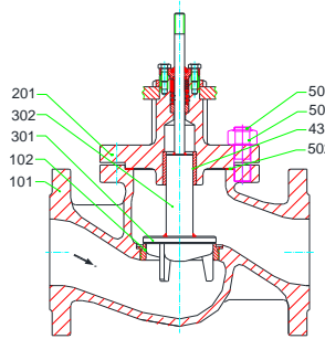
MV 5211, PV 6211 DN 80 – 100, PN 16 – 40
