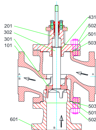
MV 5221, PV 6221 DN 100, PN 16 – 40
