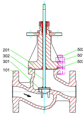
MV 5211, PV 6211 DN 15 – 50, PN 63 – 160
