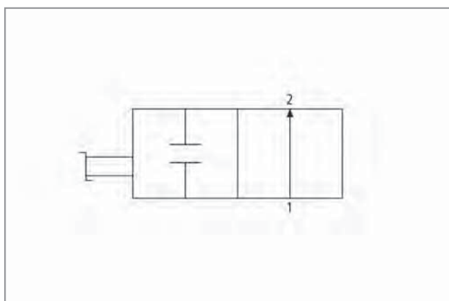
Функциональная схема KVZ (1 = вакуумный генератор; 2 = присоска)
